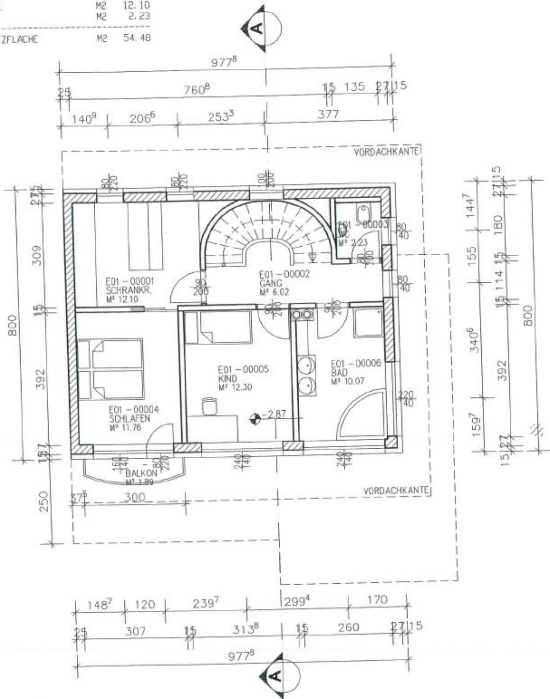
OBERGESCHOSS 1:100
