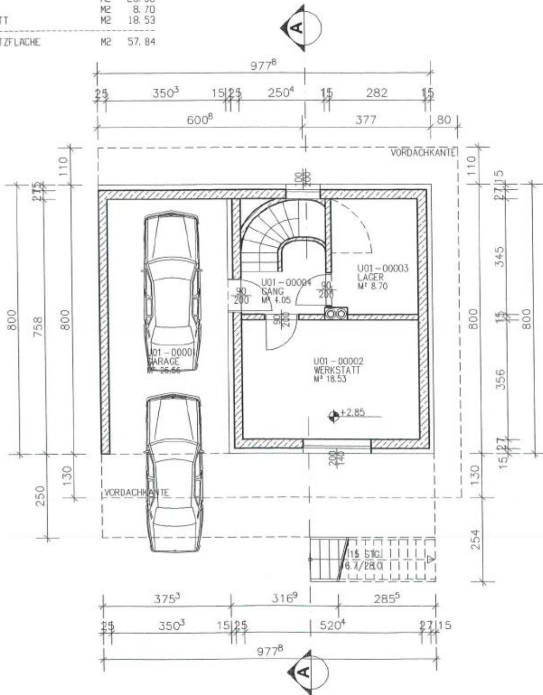
KELLERGESCHOSS 1:100
