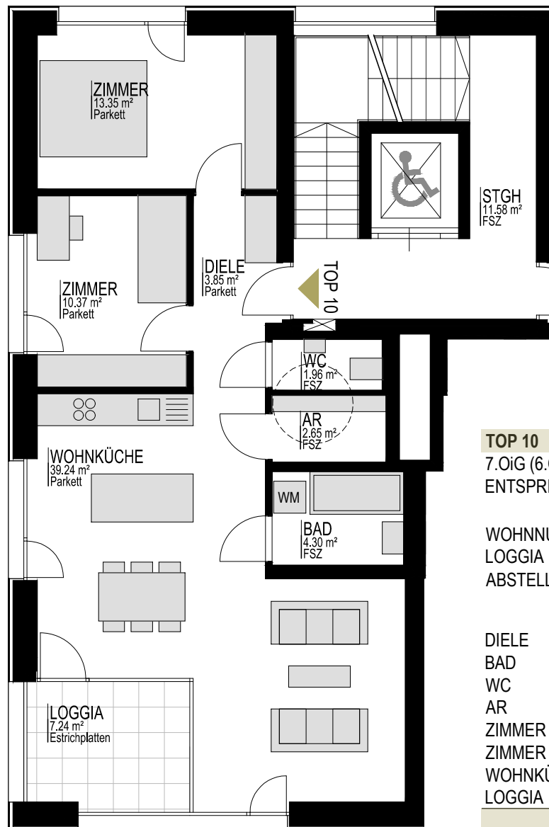
GRUNDRISS M 1:100
