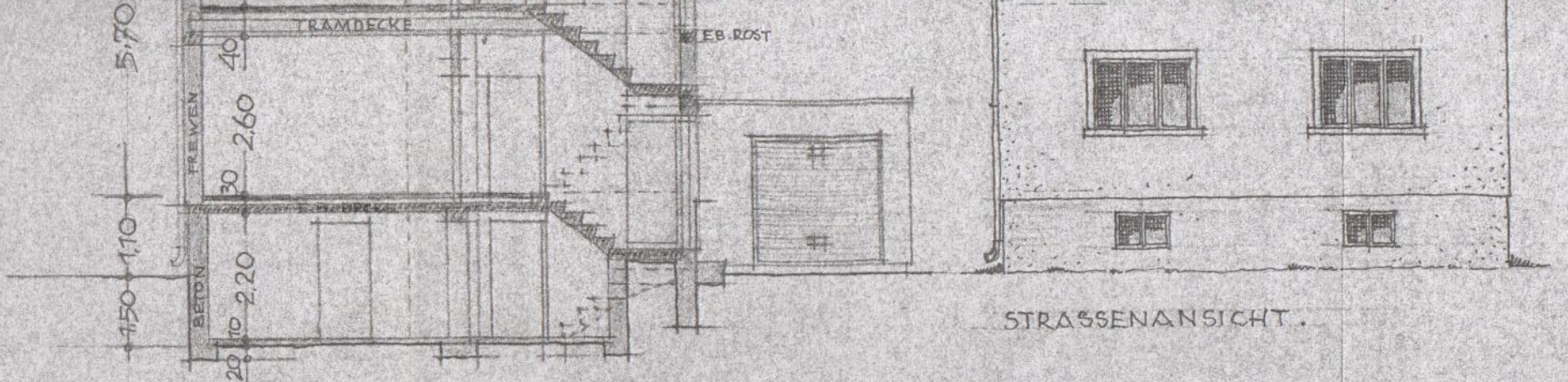
SCHNITT: A-B.
