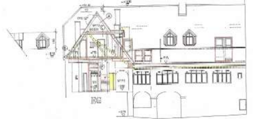
ANSICHT 05W - 59W SCHEMATA 002B
