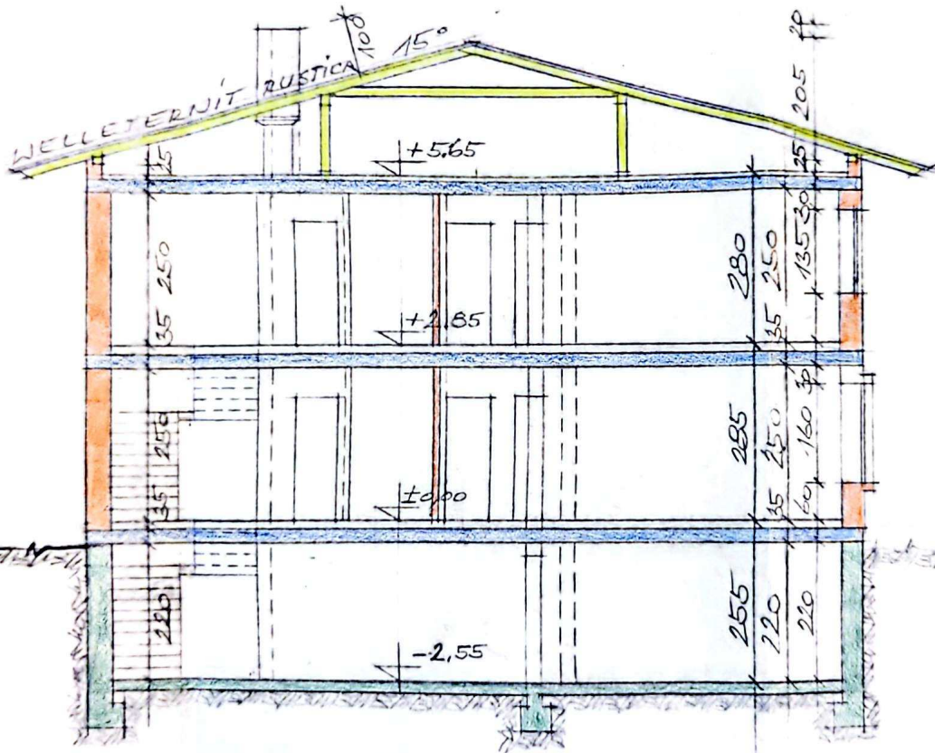
SCHNITT
